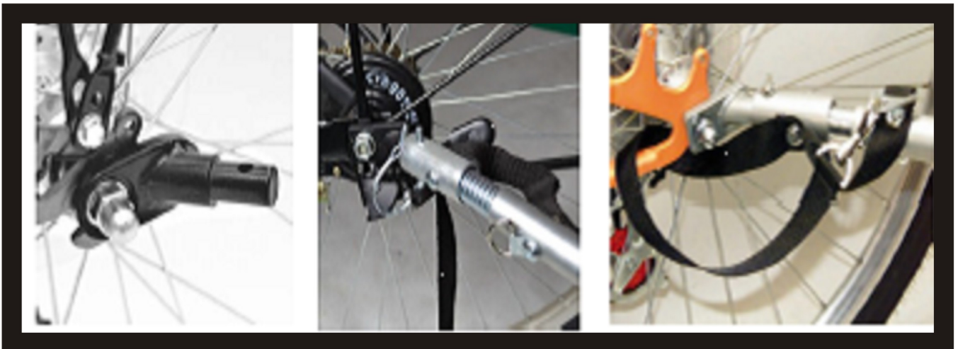
EL ACOPLE SE AJUSTA AL EJE DE LA BICICLETA, QUEDANDO FIJO EN POSICION HORIZONTAL, PERMITIENDO ACOPLAR Y DESACOPLAR EL CARRITO A LA BICICLETA. LA CORREA DE SEGURIDAD SE PUEDE ENGANCHAR AL CUADRO O SIMPLEMENTE ENROSCARLA EN LA BARRA PARA QUE NO QUEDE SUELTA
