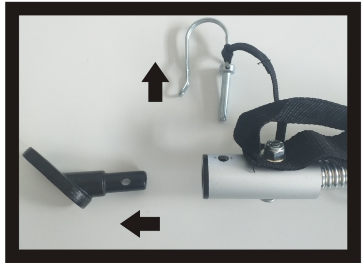
RETIRAR EL ACOPLE NEGRO DEL EXTREMO DE LA BARRA QUITANDO EL PASADOR
